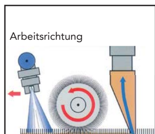
Funktionsweise der Powerwalze
