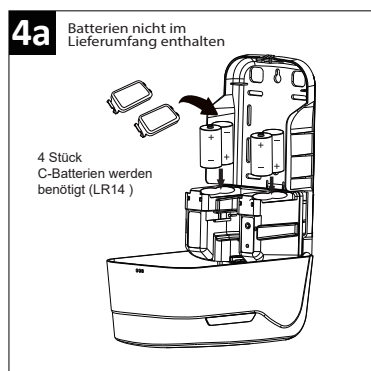
Legen Sie die Batterien in die beiden Batteriefächer
